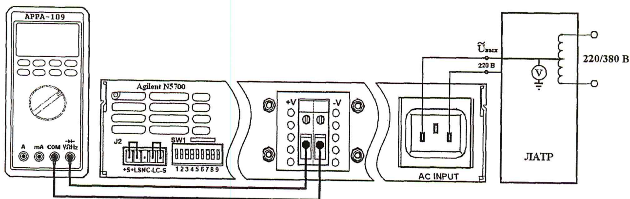
Рисунок 1 Структурная схема соединения приборов для определения абсолютной погрешности установки напряжения постоянного тока, определения нестабильности выходного напряжения постоянного тока при изменении напряжения электропитания источника, где:
