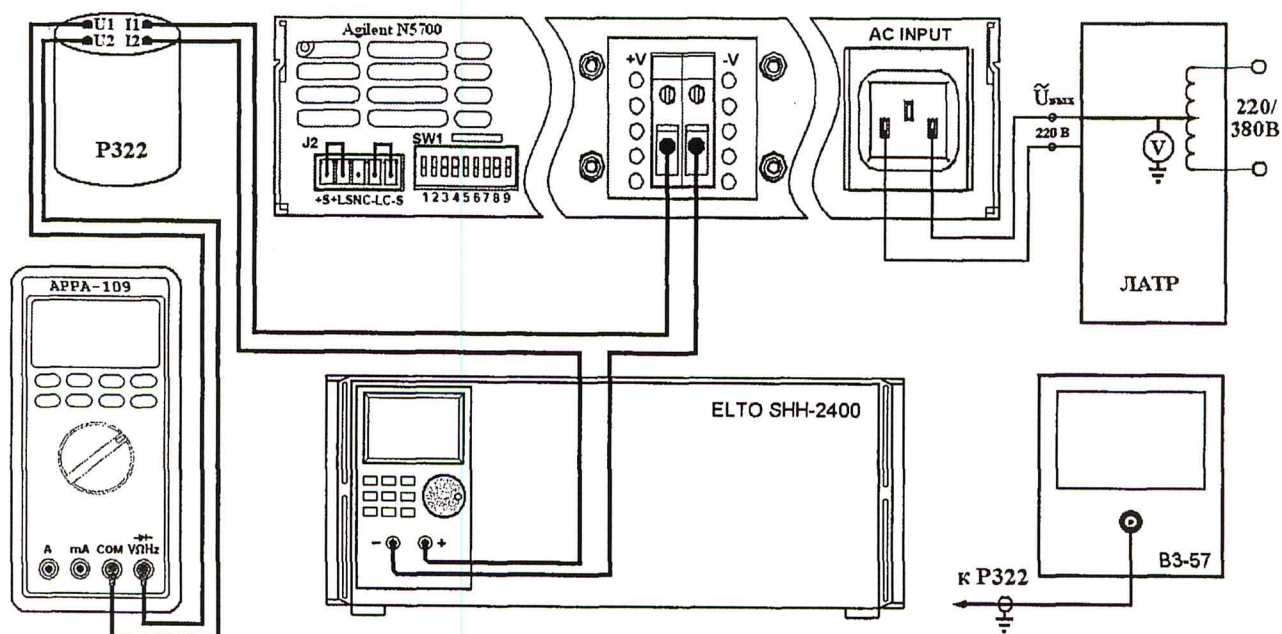
Рисунок 3 Структурная схема соединения приборов для определения метрологических характеристик источников питания в режиме стабилизации тока, где:
