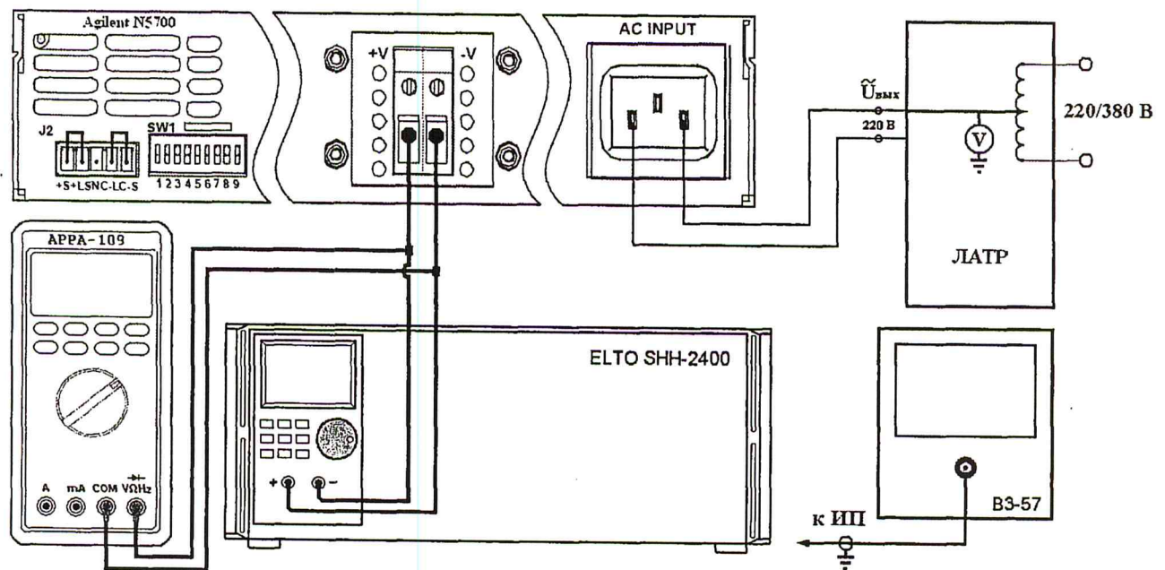
Рисунок 2 Структурная схема соединения приборов для определения нестабильности выходного напряжения постоянного тока при изменении тока нагрузки, определения уровня пульсаций выходного напряжения постоянного тока, где:
