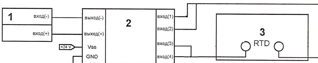
1 – модуль аналогового ввода; 2 – барьер искробезопасности; 3 – многофункциональный калибратор/магазин сопротивлений; Рисунок А.5 – Схема соединения приборов при поверке входных аналоговых измерительных каналов температуры с помощью термопреобразователей температуры
