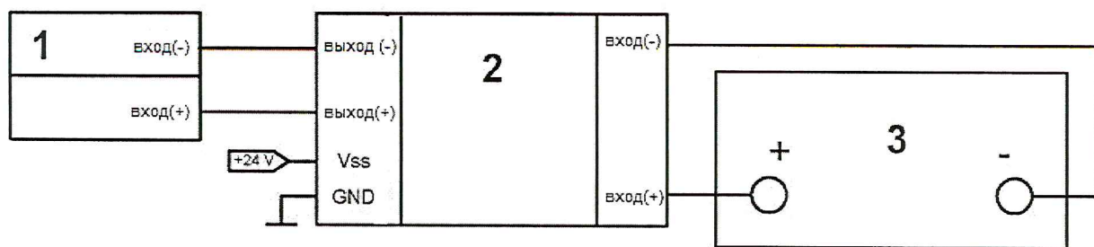
1 – модуль аналогового ввода; 2 – барьер искробезопасности; 3 – многофункциональный калибратор; Рисунок А.4 – Схема соединения приборов при поверке входных/выходных аналоговых измерительных каналов типа «4 – 20 мА униполярный» в составе с промежуточными измерительными преобразователями с гальванической развязкой (барьерами искробезопасности)
