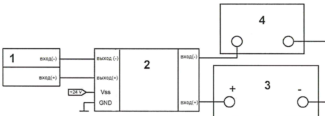
1 – модуль аналогового ввода; 2 – барьер искробезопасности; 3 – многофункциональный калибратор; 4 – магазин сопротивлений; Рисунок А.3 – Схема соединения приборов при поверке входных аналоговых измерительных каналов типа «4 – 20 мА униполярный» в составе с промежуточными измерительными преобразователями с гальванической развязкой (барьерами искробезопасности)
