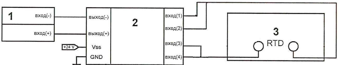
1 – модуль аналогового ввода; 2 – барьер искробезопасности; 3 – многофункциональный калибратор/магазин сопротивлений; Рисунок А.5 – Схема соединения приборов при проверке входных аналоговых измерительных каналов температуры с помощью термопреобразователей температуры
