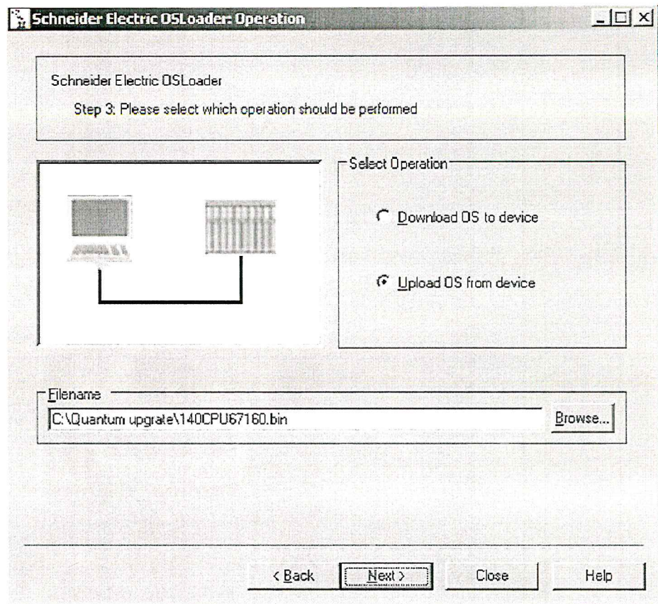
Рисунок 2 – Выбор операции
