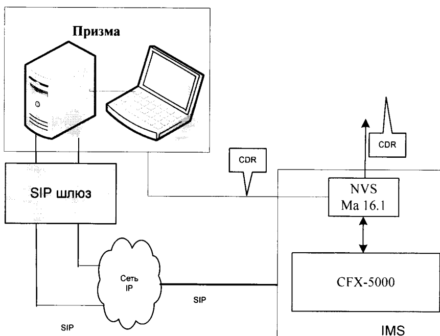
Рисунок 1- Схема поверки
