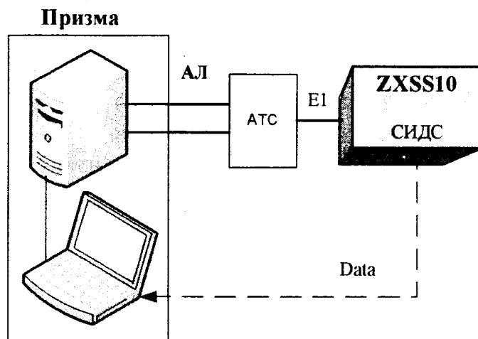
Рисунок 2 - Схема поверки СИДС (через промежуточную АТС)
