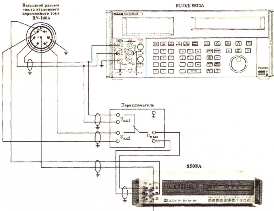
Рисунок 1 – Структурная схема проверки погрешности воспроизведения коэффициента преобразования
