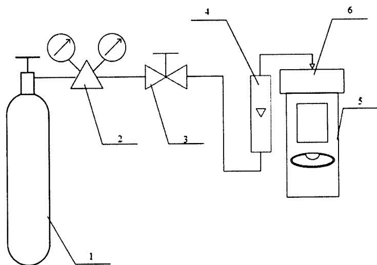
Рисунок 1 – Схема подачи ПГС в ИК системы измерительной газоаналитической RAE Systems модели Meshguard
