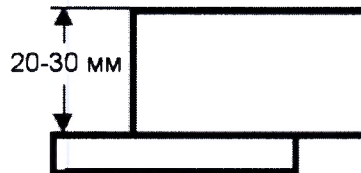
Рисунок 1 - Ступенька из концевых мер длины для определения абсолютной погрешности измерений по оси Z
