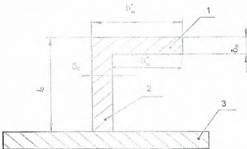
Рисунок А.13 – Рамный набор (отфланцовый профиль).
