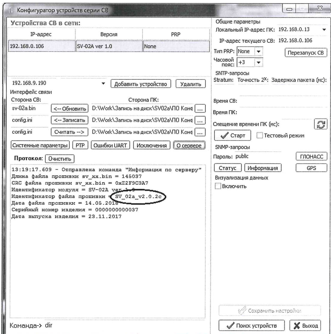
Рисунок 7 – Идентификация ПО.
