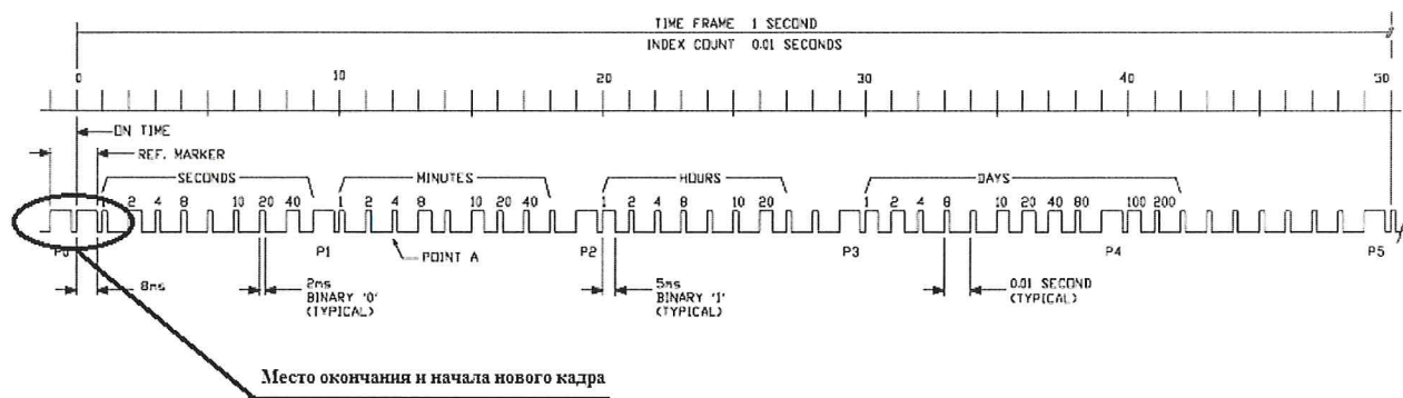
Рисунок 5 – Структура телеграммы IRIGB-007
