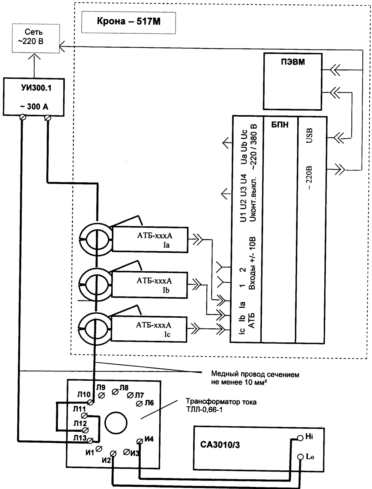
Рисунок А.4 Схема подключения стенда при определении погрешности измерений силы переменного тока на пределе 100 А
