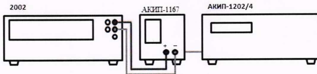
Рисунок 1 – Схема соединения приборов при определении погрешности воспроизведения напряжения постоянного тока
