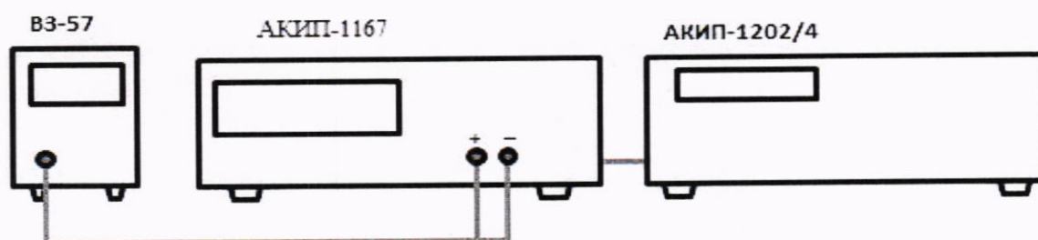
Рисунок 3 – Схема соединения приборов при определении уровня пульсаций выходного напряжения
