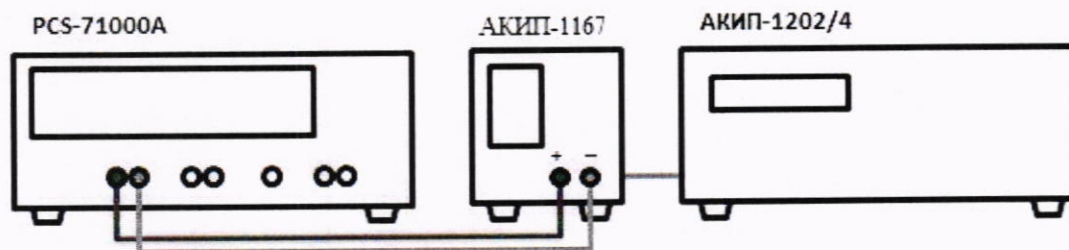
Рисунок 4 – Схема соединения приборов при определении погрешности воспроизведения силы тока
