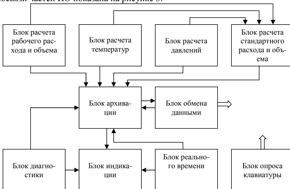
Рисунок 3 - Структура ПО
