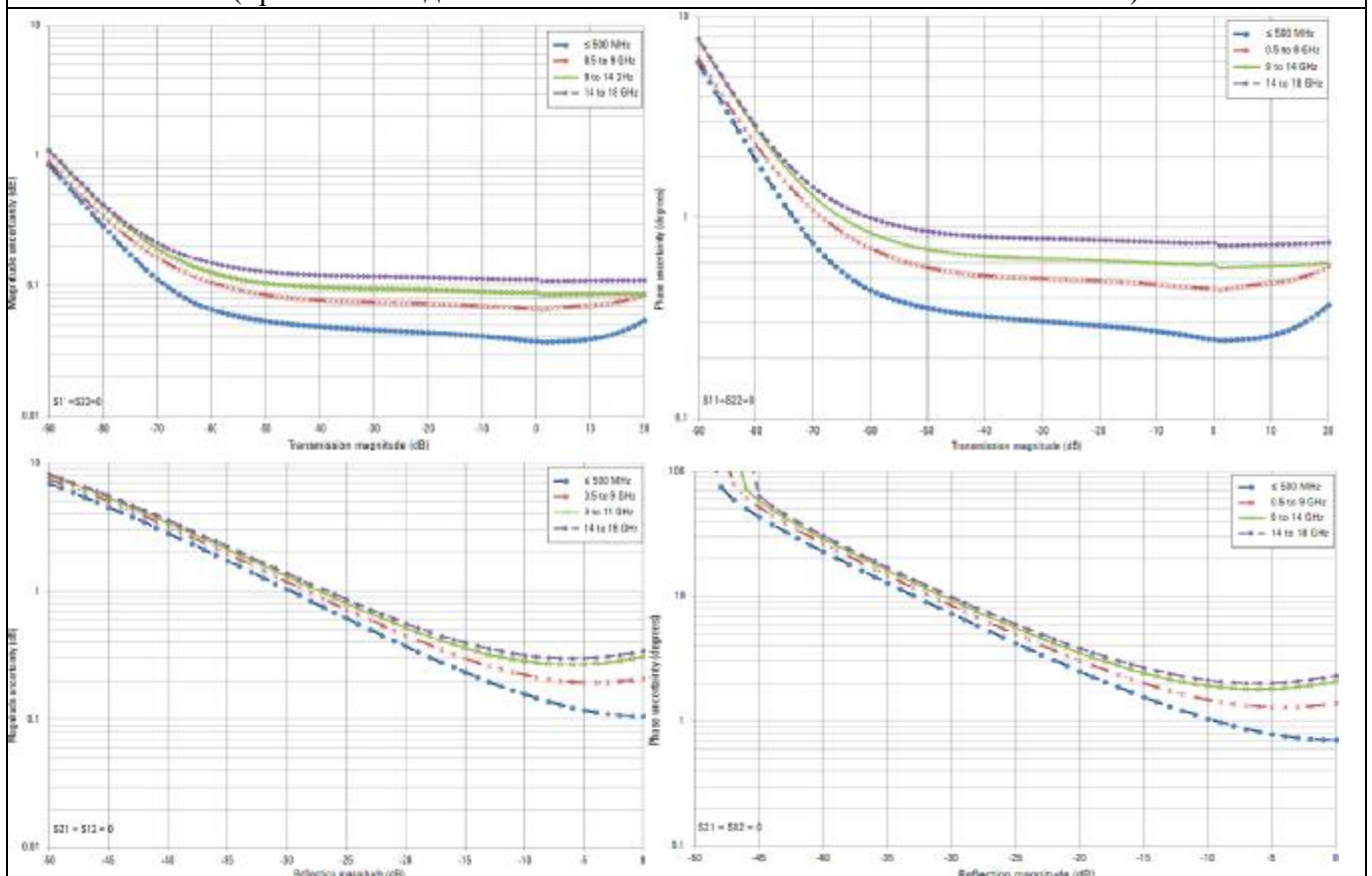
Погрешность коэффициентов передачи и отражения (амплитуда и фаза) (заводские установки) (применяется для FieldFox N9913/4/5/6/7A и FieldFox N9925/6/7A)
