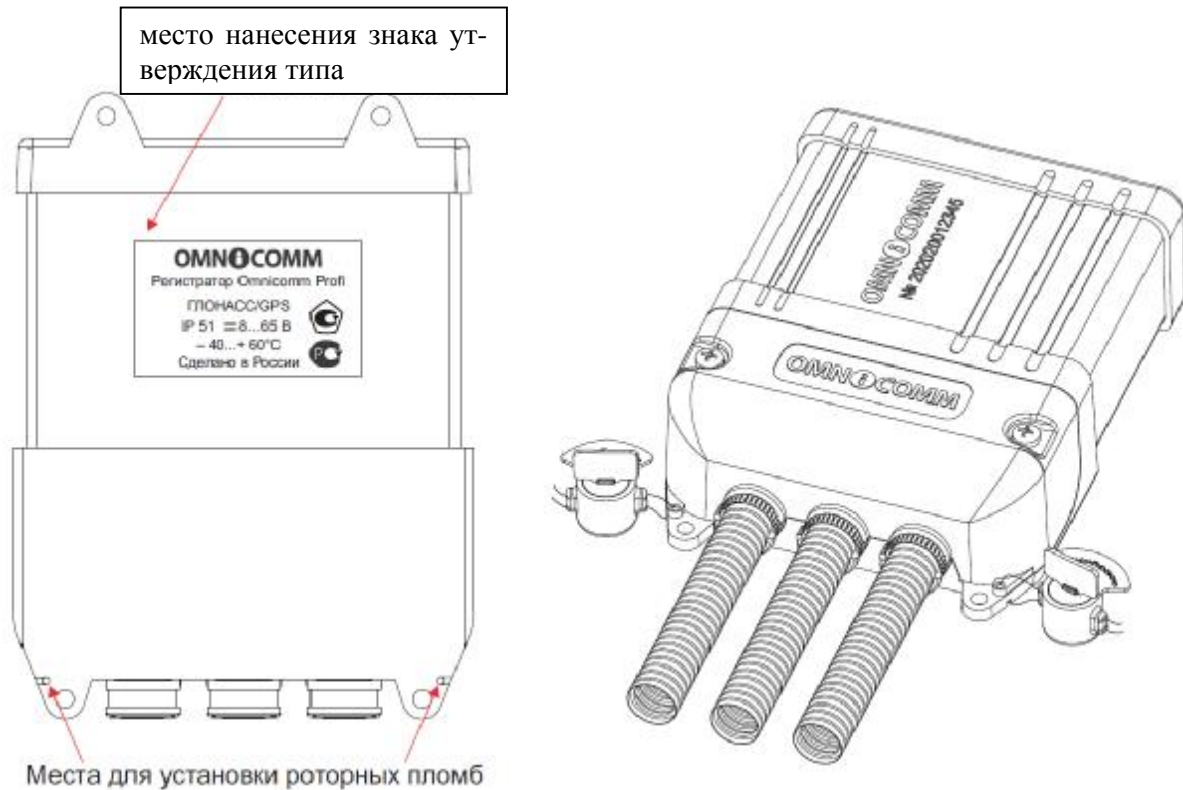
Рисунок 1 - Внешний вид аппаратуры Omnicomm Profi
