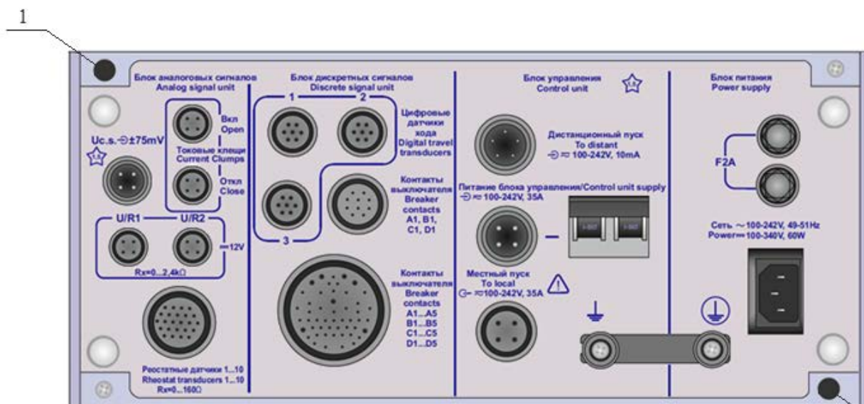
Рисунок 2 - Схема пломбировки от несанкционированного доступа (задняя панель измерительного блока ПКВ/УЗ.0) 1 - места нанесения оттисков пломб
