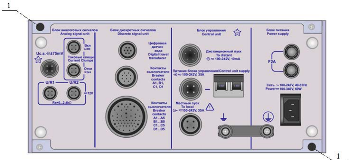
Рисунок 3 - Схема пломбировки от несанкционированного доступа (задняя панель измерительного блока ПКВ/У3.1) 1 - места нанесения оттисков пломб
