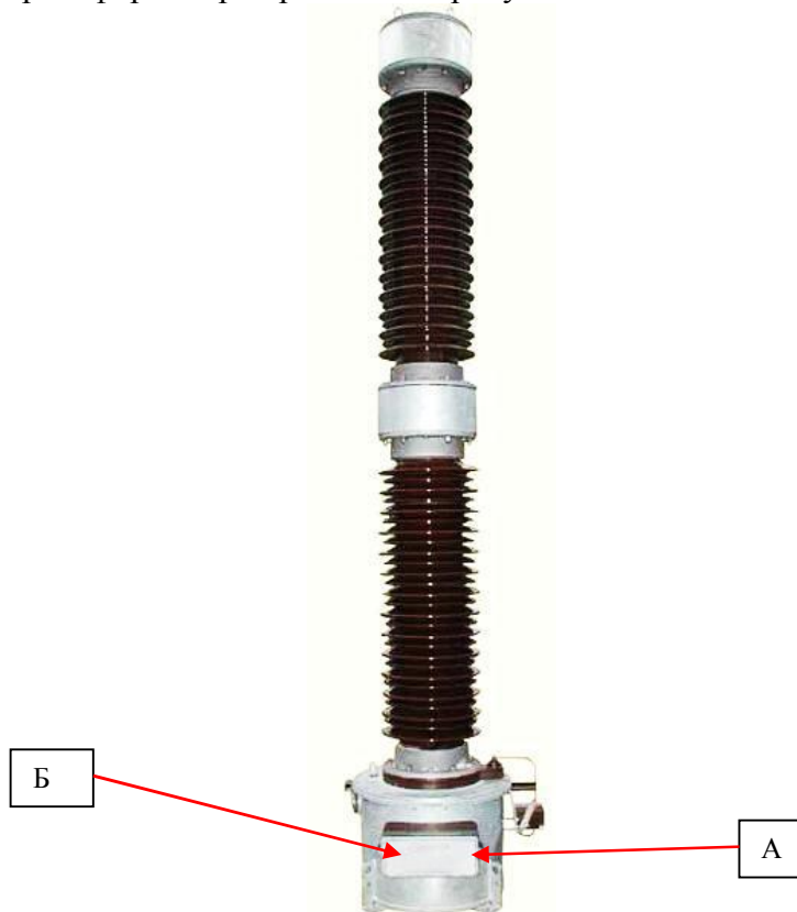
Рисунок 1 – Общий вид трансформатора напряжения емкостного DFK-245 Место пломбировки от несанкционированного доступа (А) и нанесения знака поверки (Б)
