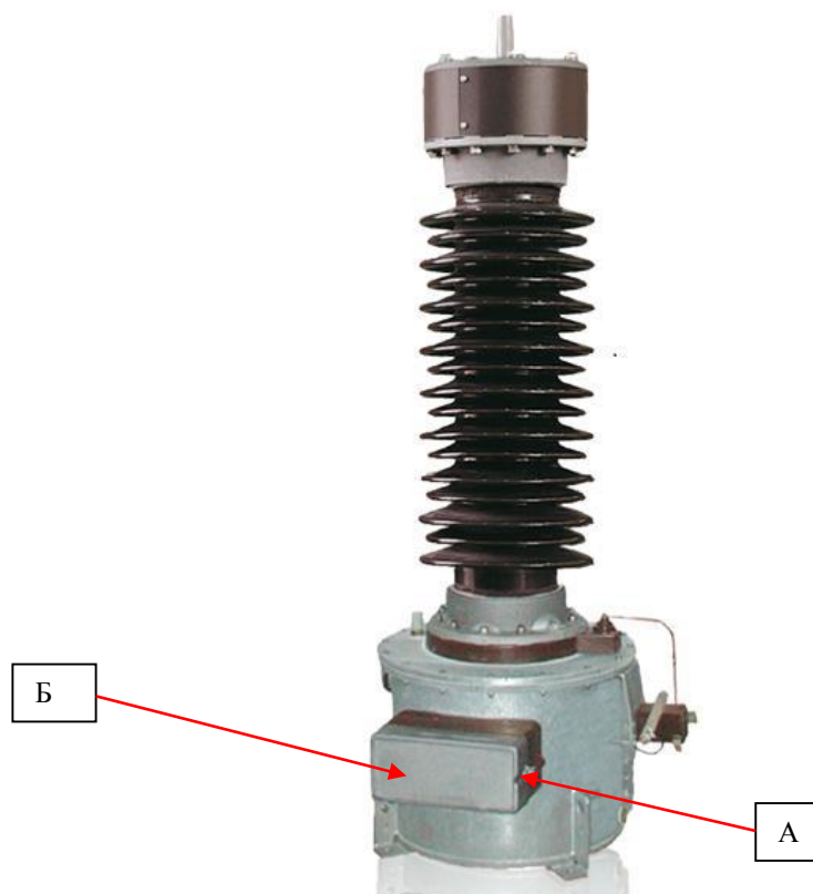
Рисунок 1 – Общий вид трансформатора напряжения емкостного DDB-123 Место пломбировки от несанкционированного доступа (А) и нанесения знака поверки (Б)
