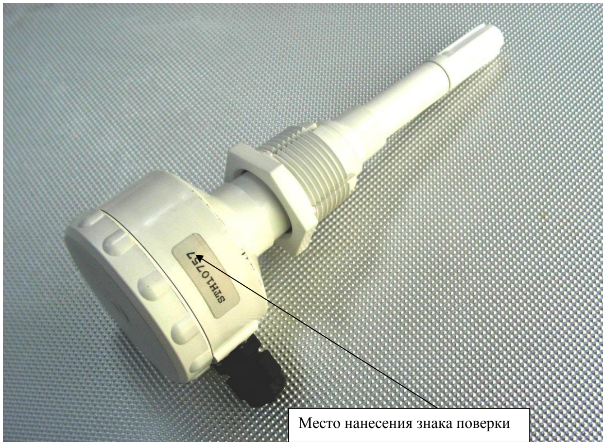
Рисунок 1 - Общий вид средства измерений и место нанесения знака поверки
