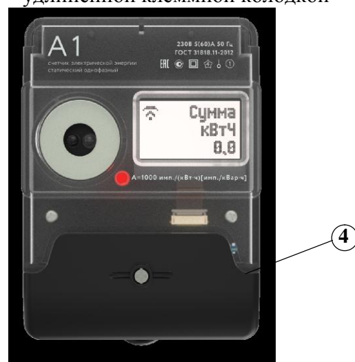
в) счетчики в корпусе «мини» с удлиненной клеммной колодкой
