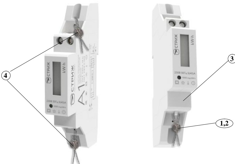
е) счетчики в корпусе «нано»
