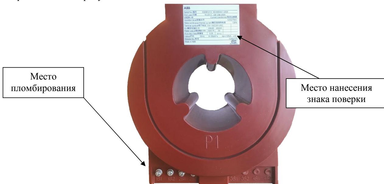
Рисунок 1 – Внешний вид трансформаторов, места пломбирования и нанесения знака поверки
