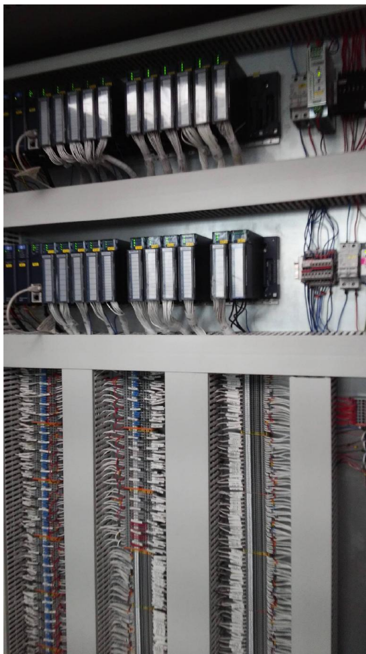
Рисунок 2 - Внешний вид модулей серии RX3i в шкафу
