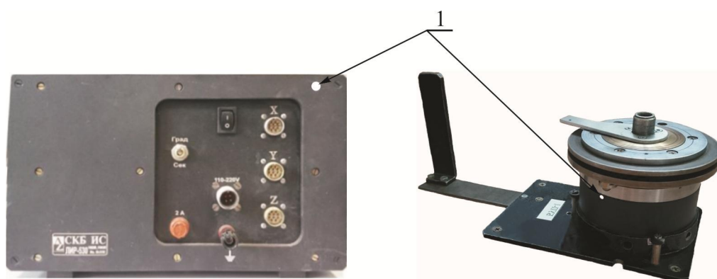
Рисунок 4 - Схема пломбировки от несанкционированного доступа 1 - места нанесения пломб
