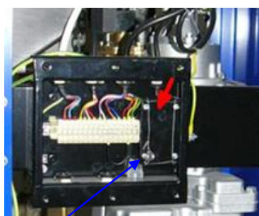
Пломба для нанесения знака поверки
