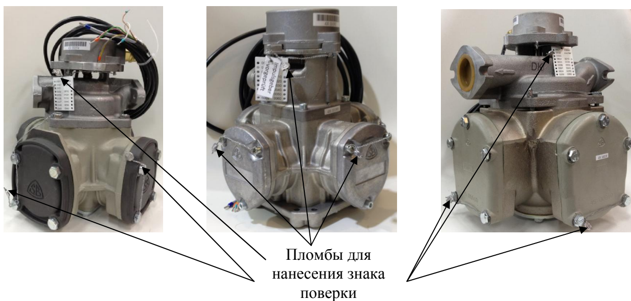
Измеритель объема КМ 0
