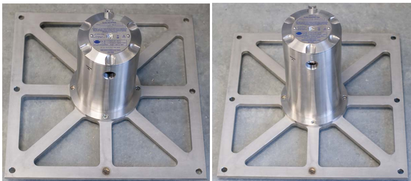
в) блок приемника и передатчика газоанализатора исполнения Senscient ELDS 1000 XD, XC на монтажной пластине
