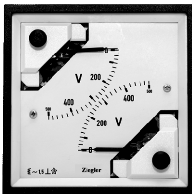
д) амперметры и вольтметры серии EQ модификации 2EQ Рисунок 1 - Внешний вид амперметров и вольтметров серий EQ, PQ и DSL
