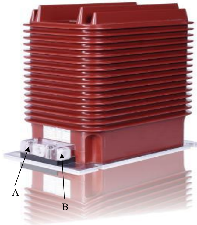
Рисунок 1 - Общий вид средства измерений и обозначение места пломбировки от несанкционированного доступа (А) и места нанесения знака поверки (Б)
