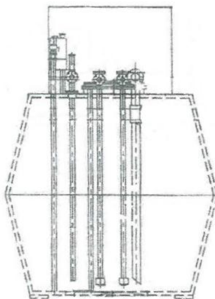
Рисунок 1 – Эскиз резервуаров РГС-10
