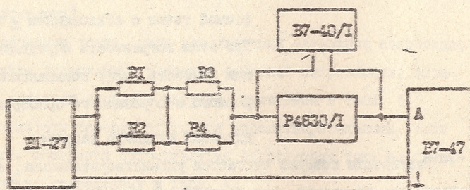
Схема поверки
