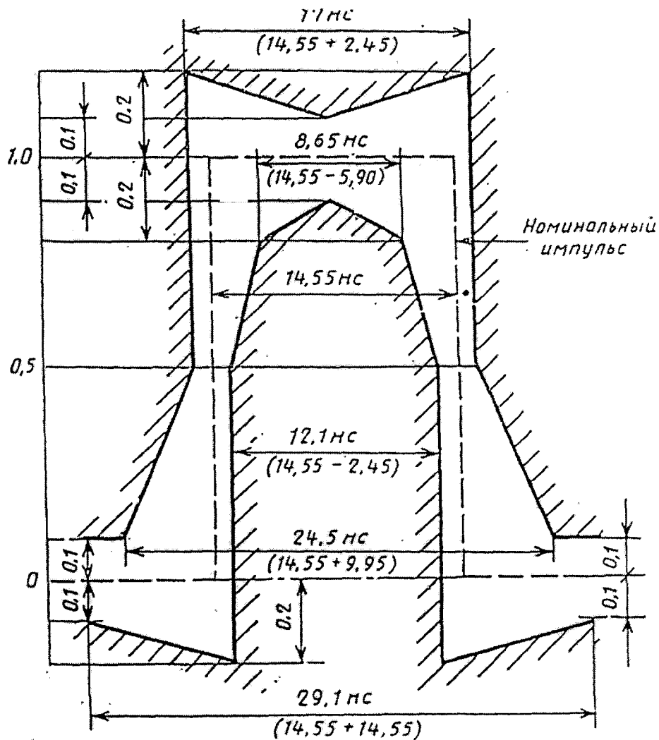
Рис.8.5. Маска формы импульса на несимметричном выходе, HDB3, 34368 Кбит/с.
