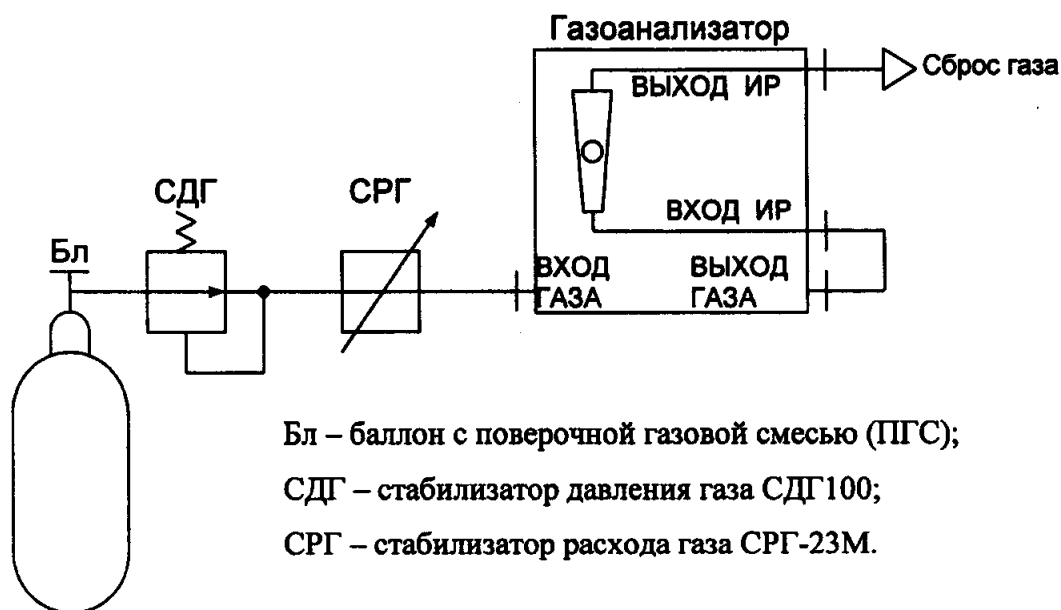
Рисунок В.2- Пневматическая схема для определения основной приведённой погрешности
