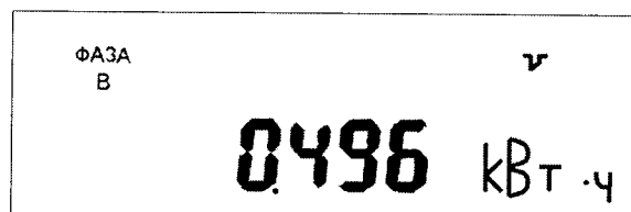
Рисунок Е.9 – Пример индикации значения суммарного потребления активной энергии по всем тарифам по фазе «В».
