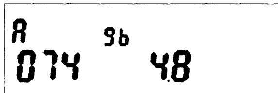
Рисунок Е.2 – Пример индикации параметров связи по интерфейсу RS-485 (адрес в магистрали RS-485 – 074, скорость обмена 4,8 кБод, режим 9- битной передачи данных)
