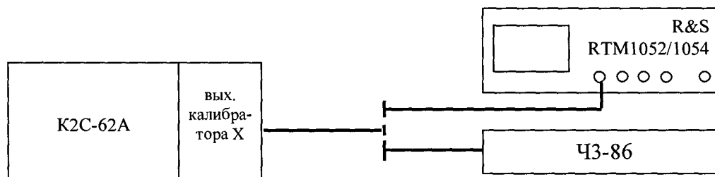
Рисунок 2 - Схема определения погрешности по частоте внутреннего опорного генератора
