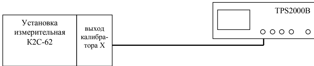
Рисунок 3– Схема определения диапазона установки коэффициентов развертки и погрешности частоты опорного генератора
