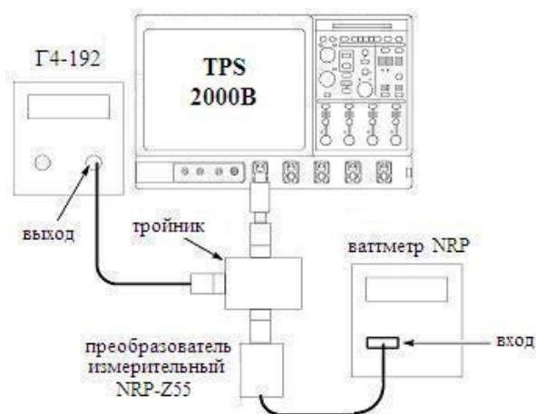
Рисунок 2б - Схема определения полосы пропускания
