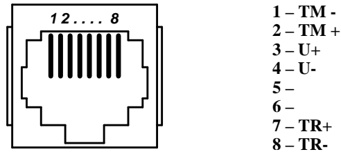
Рисунок Г.1 – Цоколевка розетки разъема электрического испытательного выхода ТМ, интерфейса RS-485 (розетка TJ2-8P8C)
