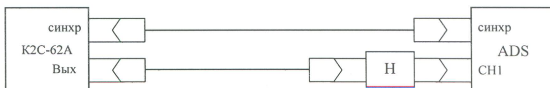
Рис. 5. Структурная схема соединения приборов для измерения времени нарастания переходной характеристики.
