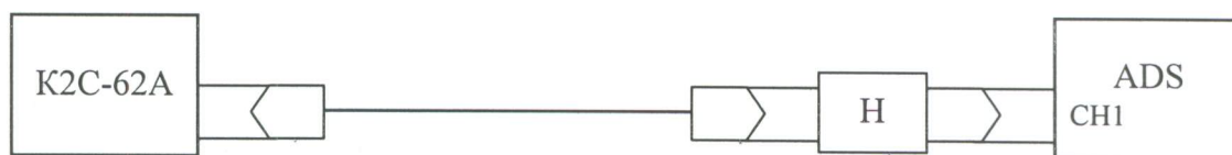
Рис. 3. Структурная схема соединения приборов для определения относительной погрешности коэффициентов развертки.
