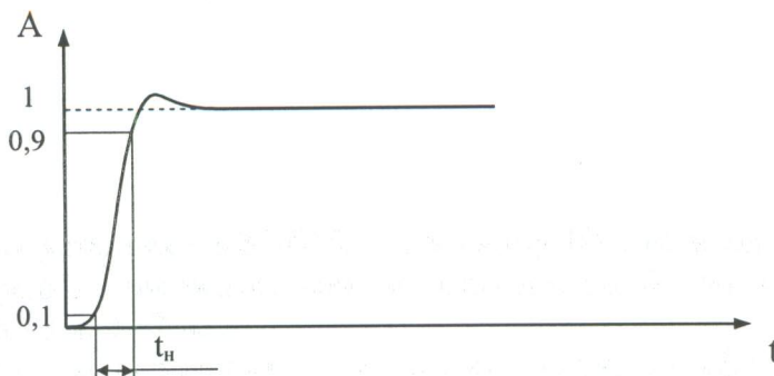
Рис. 6. Изображение испытательного импульса при измерении времени нарастания переходной характеристики t_n .
