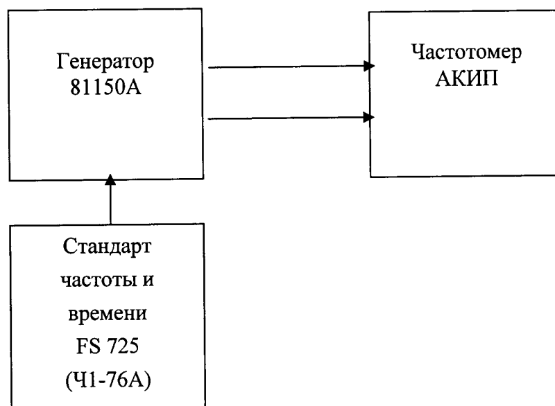
Рисунок 3 – Схема определения абсолютной погрешности измерения длительности импульсов и интервалов времени
