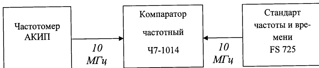
Рисунок 1 – Схема определения относительной погрешности по частоте кварцевого опорного генератора
