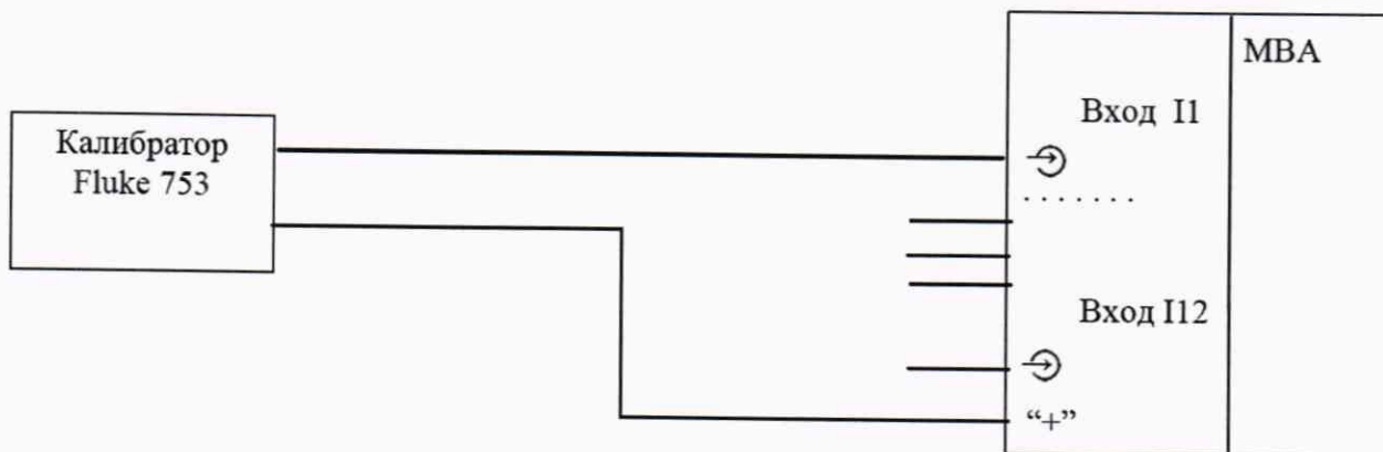
Рисунок 2 - Схема подключения для определения погрешности измерений силы постоянного тока по измерительным каналам модуля МВА для ПТК шкафных исполнений У1 и У3
