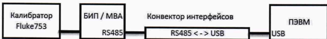
Рисунок 1 - Схема подключения для опробования и подтверждения соответствия программного обеспечения
