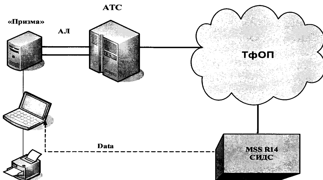
Рисунок 1 - Схема поверки СИДС по аналоговым абонентским линиям
