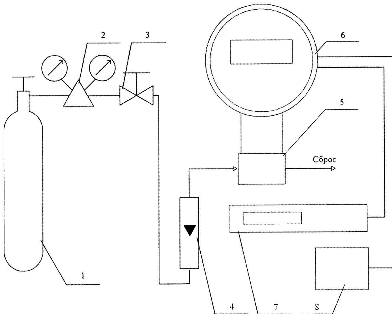
1 – источник ГС (баллон или генератор); 2 – редуктор баллонный; 3 – вентиль точной регулировки; 4 – индикатор расхода (ротаметр); 5 – адаптер поверочной газовой смеси; 6 – газоанализатор; 7 – измерительный прибор; 8 – источник питания.
