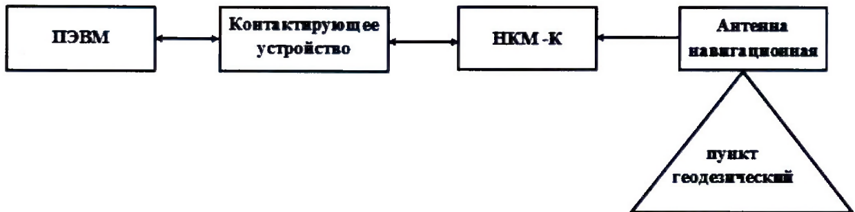
Рисунок 3 – Схема проведения измерений при определении абсолютной погрешности определения координат местоположения
