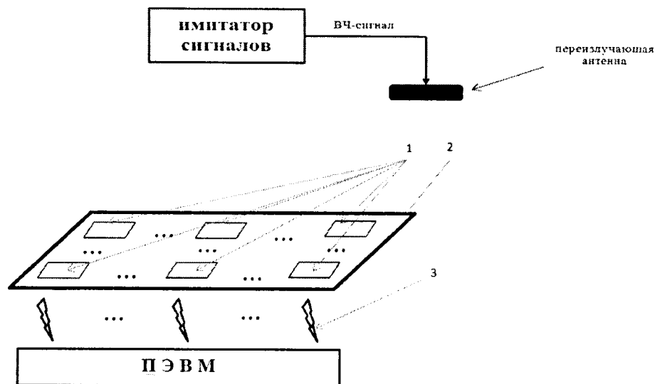
Рисунок 1 – Схема проверки работоспособности
