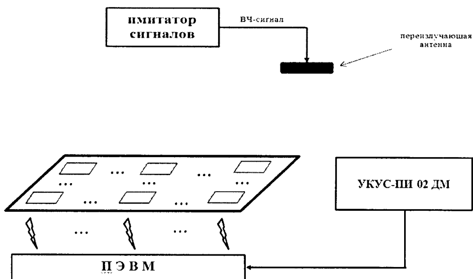
Рисунок 3 – Схема проведения измерений при первичной поверке устройства
