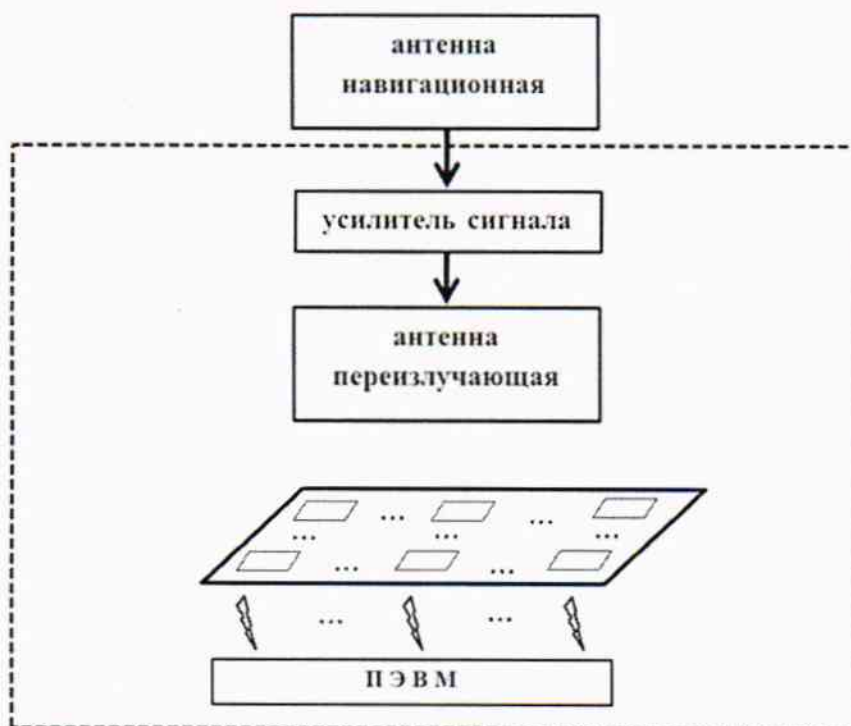
Рисунок 5 – Схема проведения измерений при определении погрешности определения координат при первичной поверке
