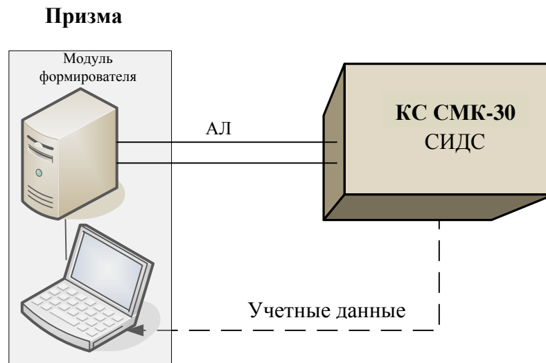
Рисунок 1- Схема поверки
