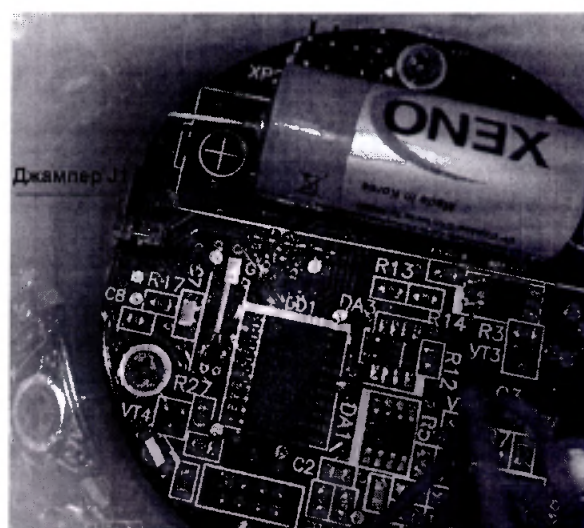
Рисунок 2 – Расположение джампера J1
