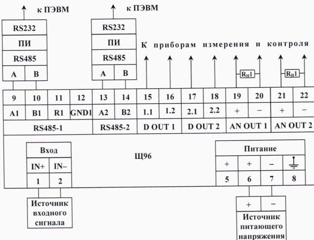
Рисунок А.2 – Схемы подключения приборов Щ72
