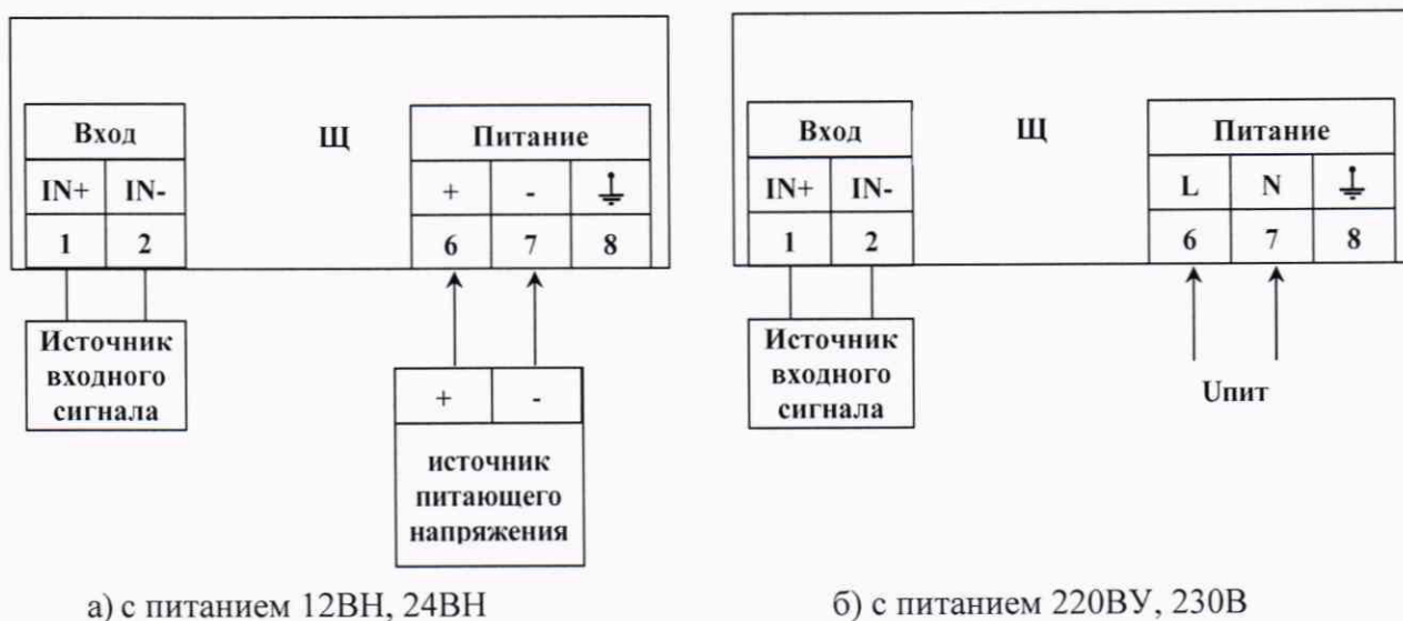
Рисунок А.4 – Схемы подключения приборов Щ120
