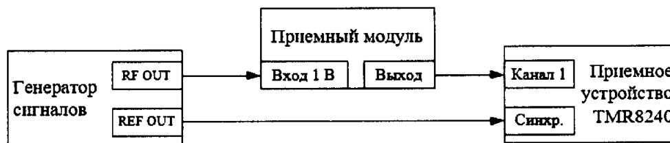
Рисунок 1 – Схема подключения
