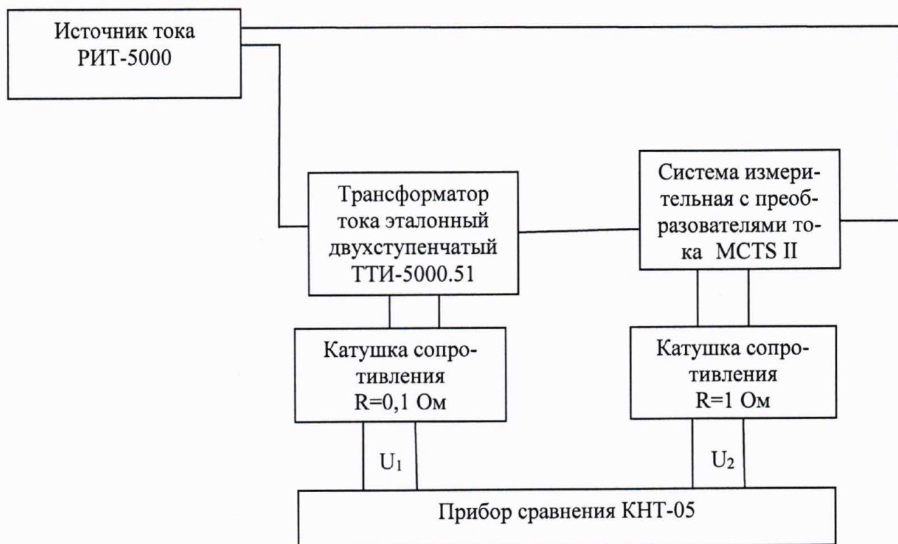
Рисунок 1 – Схема определения характеристик системы на переменном токе
