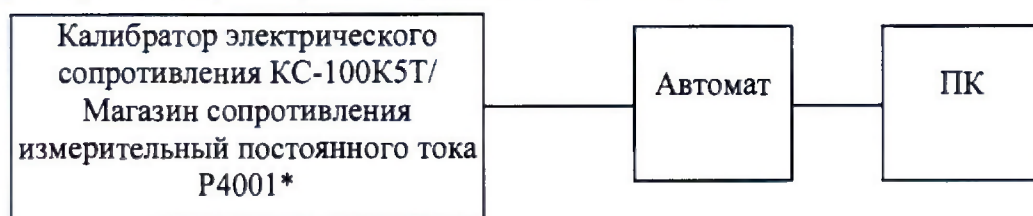
Рисунок 1 – Схема структурная определения основной относительной погрешности измерений электрического сопротивления изоляции
