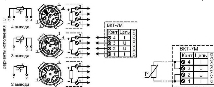
а) Подключение ТС по 4-проводной схеме
