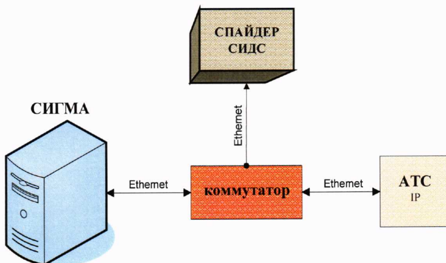
Рисунок 1- Схема поверки
